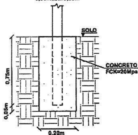
DETALHE DE FIXAÇÃO AO SOLO
